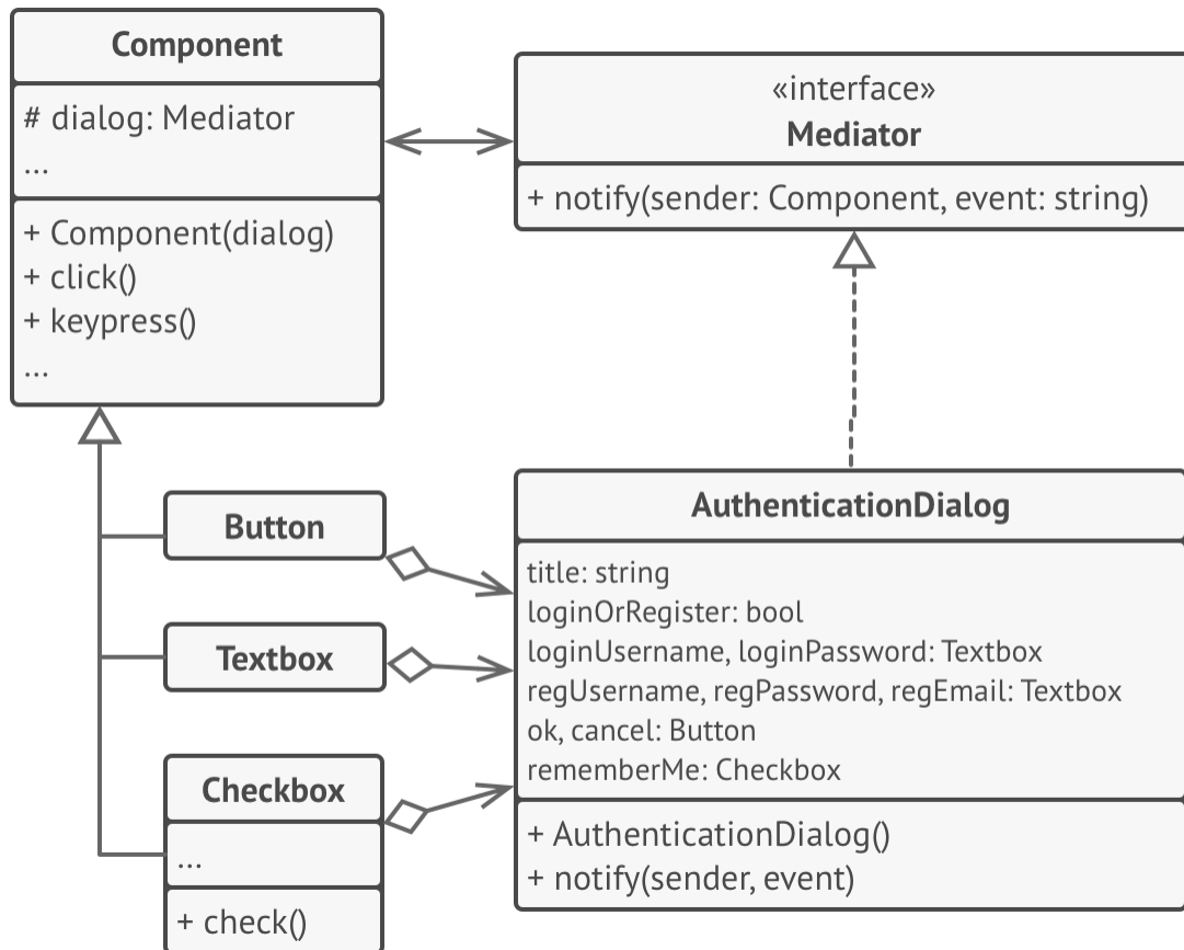
Пример структурирования классов UI-диалогов.
