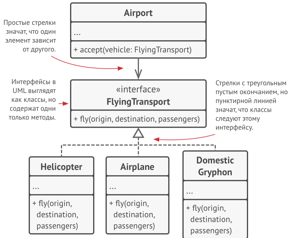
UML-диаграмма реализации и использования интерфейса.
