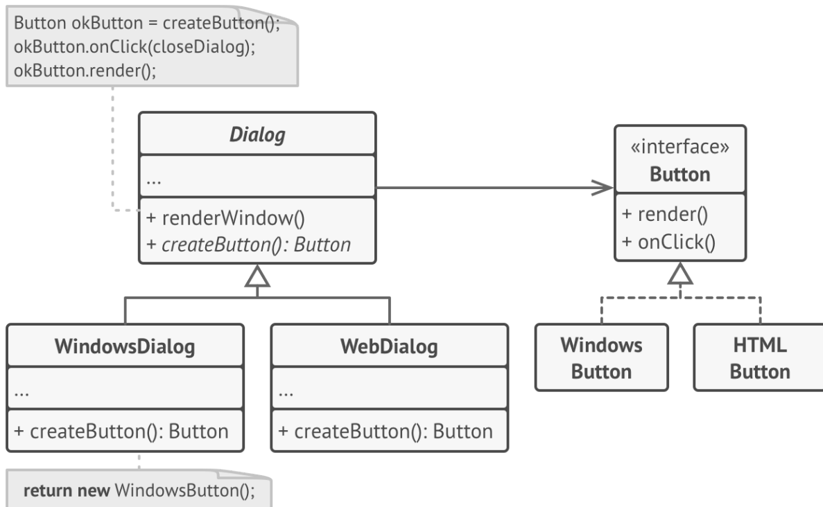
Пример кросс-платформенного диалога.
